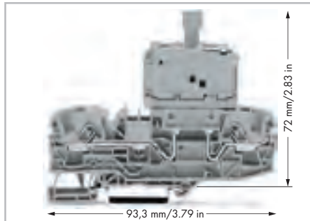
Размеры предохранительного штекера
