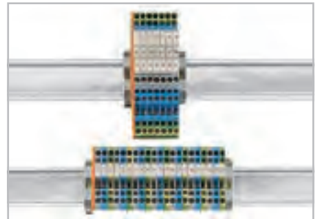
Сохраните 67% пространства рельса, используя трехуровневые клеммы.
