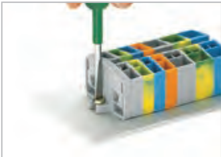
Клеммы с крепежными фланцами, винтовое крепление.
