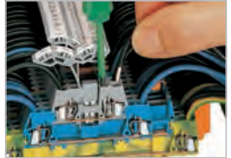
Зажим проводника
