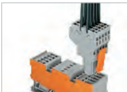
1-проводная/1-диодная базовая клемма с 2 позици- ми для перемычек 2-проводная розетка
