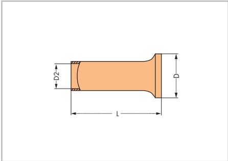
Размеры неизолирующих наконечников, см. в технических данных.
