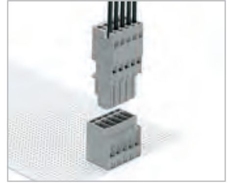
Штекерные монтажные блоки с прямыми выводами под пайку: 769-632 ... 769-645
