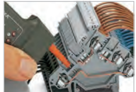
Проверка с помощью индикатора напряжения прямо на токопроводящей шине.
