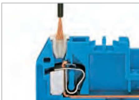
Вставьте зачищенный раскрученный проводник в изолирующий стопор.
