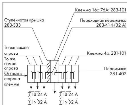
Объединение клемм от 16 мм 2 /AWG 6 (серия 283) до 4 мм 2 /AWG 12 (серия 281) для монтажа на рейку.
