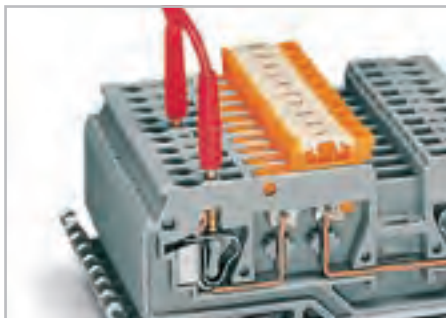
Тестовый разъем: для тестового штекера 2 мм Ø или 2,3 мм Ø – с прямым подключением к токопроводящей шине.
