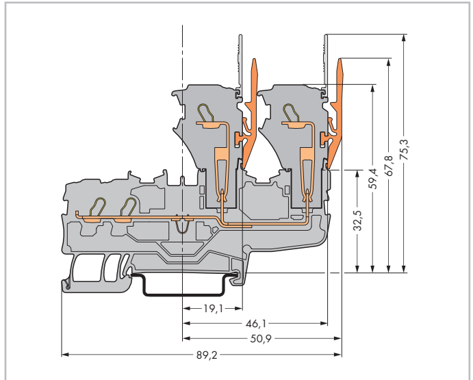
Базовая клемма с двумя 1-проводными розетками
