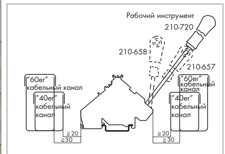
Мин. дистанция монтажа - длина провода от клемм до кабеля
