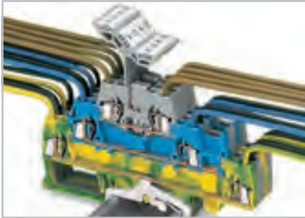
3-проводная разводка с дополнительным фазным отводом.
