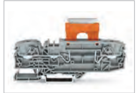
Оранжевый штекерный размыкатель (2006-8401) в исходном положении
