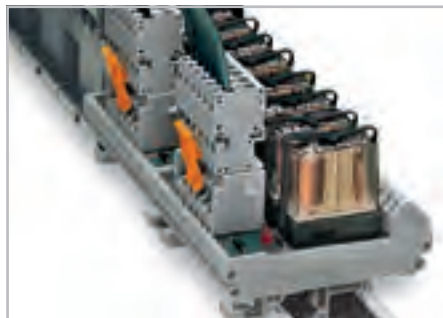
В примере использования показан модуль реле: Штекеры с прямыми выводами под пайку и 1-проводные розетки.
