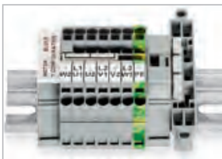
Эта перемычка разработана специально для соединений по схеме «звезда» и используется на клеммной панели электродвигателей, оснащенных монтируемыми на DIN-рейку клеммами TOPJOB® S.
