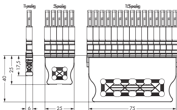
Размеры пластины фиксатора
