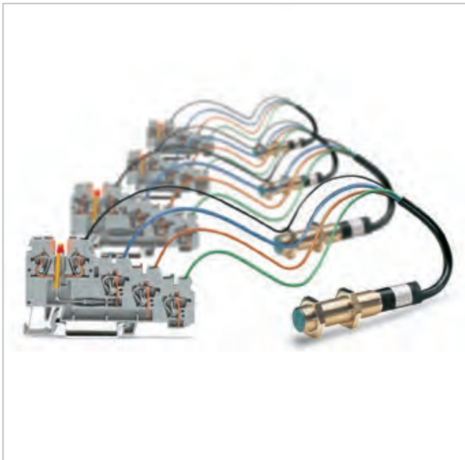
Объединение по напряжению уровня сигнала с помощью изолированных гребешковых перемычек серии 870, 2... 9-контактов, в зависимости от применения. Клеммы для датчиков со светодиодом не могут быть объединены по уровню сигнала.
