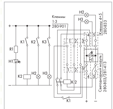
Устройство управления
