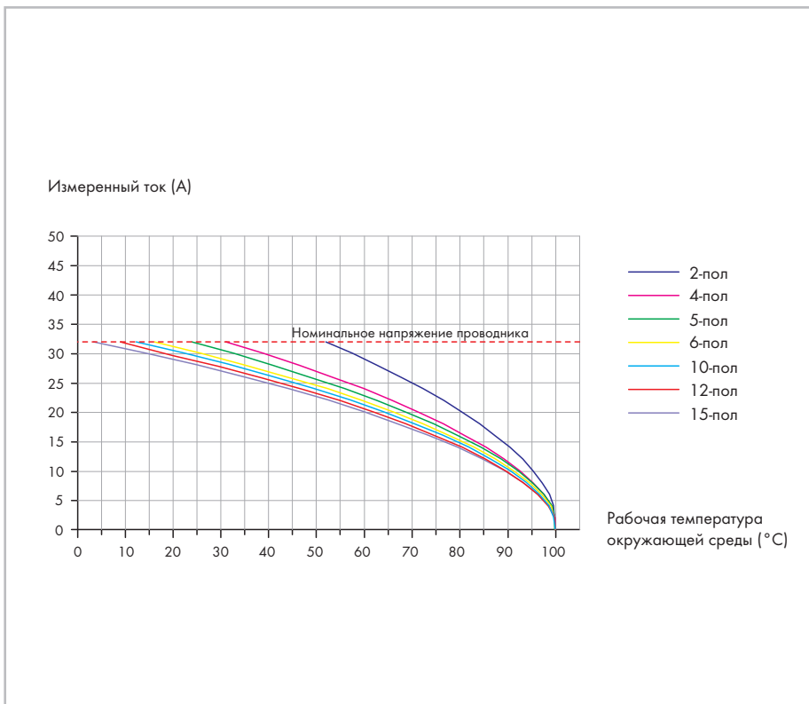
4-конт. базовые клеммы: 769-151
