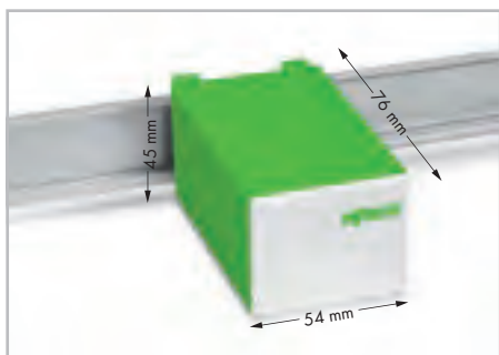
Габариты в мм Высота от верхнего края DIN-рейки 35 мм
