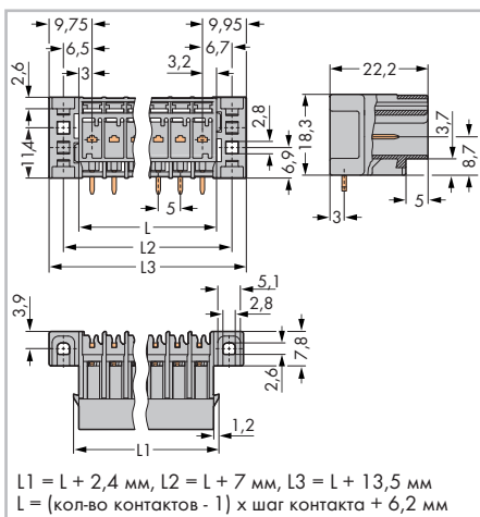
Штекер и 1-проводная розетка с фиксирующими рычагами.
