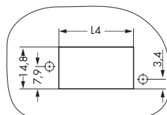
Отверстия для фиксирующих рычагов с одним контактом
