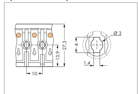
Внимание! Максимальный диаметр резьбы для самонарезающих винтов: 3,0 мм
