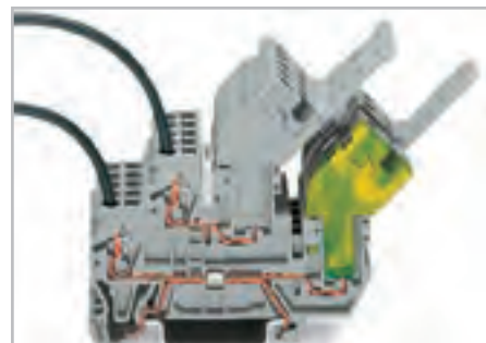
Розетки углового исполнения обеспечивают уменьшение высоты установки
