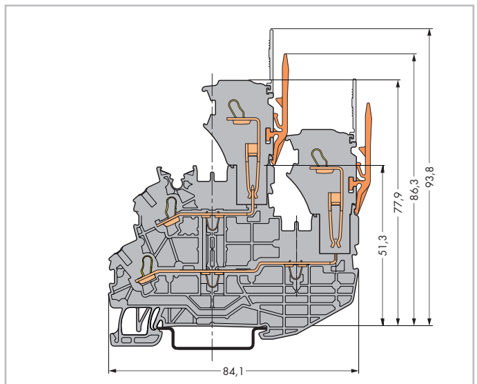
Двухуровневая базовая клемма с двумя 1-проводными розетками
