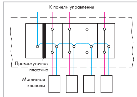
Подвод питания на стороне шкафа управления.
