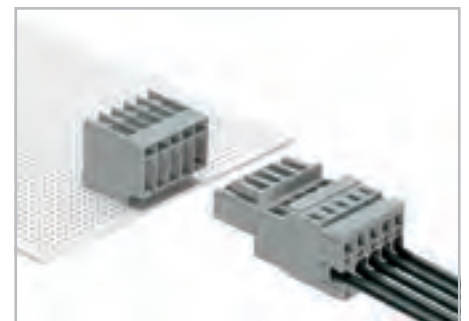
Штекерные монтажные блоки с угловыми выводами под пайку: 769-662 ... 769-675
