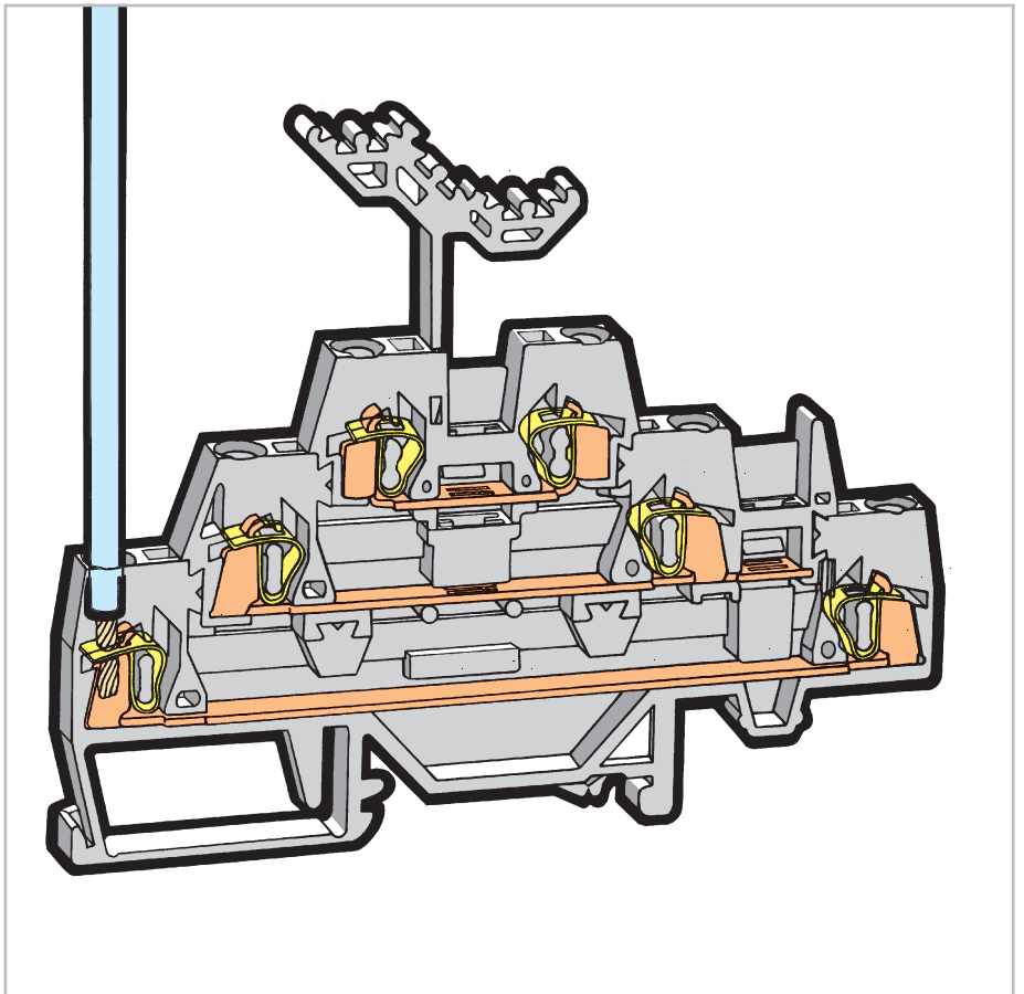
Объединение поперечными перемычками 280-402. Утопите поперечную перемычку до упора.
