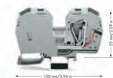
Заделка проводника 35 мм 2 /AWG 2.
