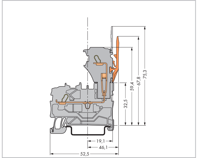
Базовая клемма с 1-проводной розеткой
