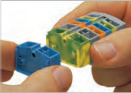
Установка модульных клемм в клеммные сборки.
